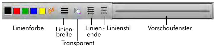
Eigenschaftsleiste
