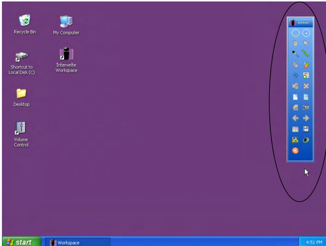
Workspacefenster - Hauptwerkzeugeiste
